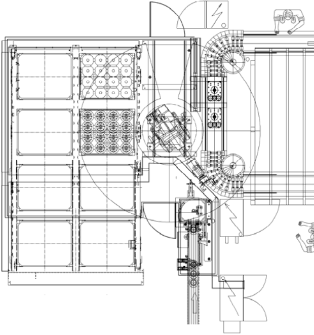
Manipulación caja diferencial
